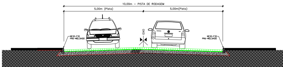
SEÇÃO TIPO DE BLOCO INTERTRAVADO - RUA II - LOT. ZANETTI
